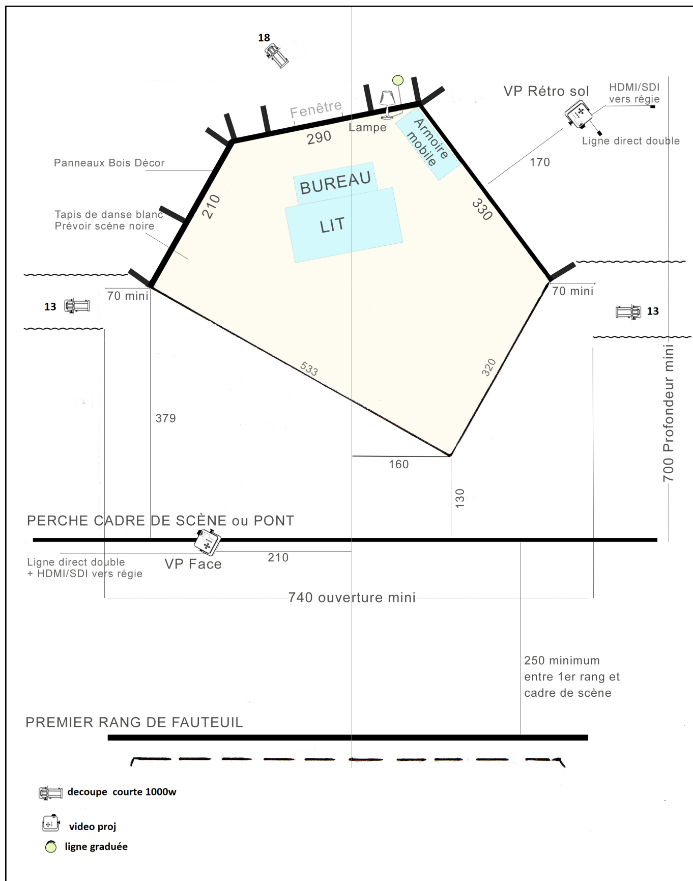
Plan de Feu Grill
